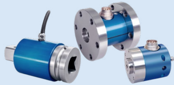
Reaktive Drehmomentsensoren, nicht rotierend
